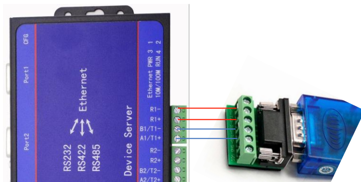
图 1.2.3 RS422（RS485）接法
