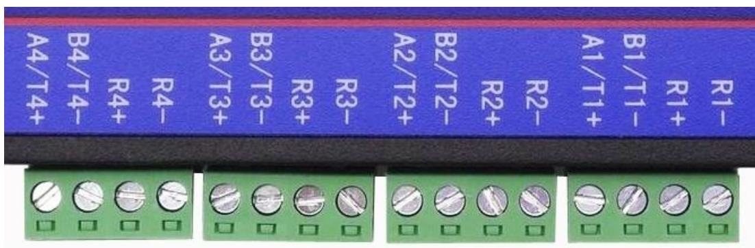
RS485/422接口定义（以第一路串口PORT1为例）
